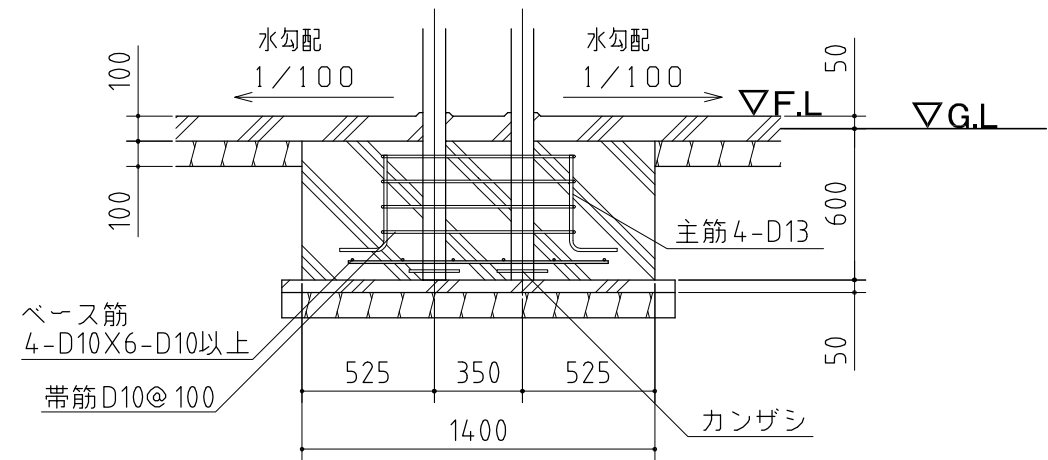
A-A' 断面
